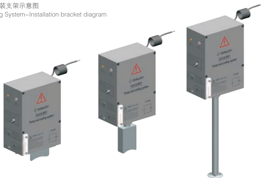
B01水冷系统-安装支架示意图
